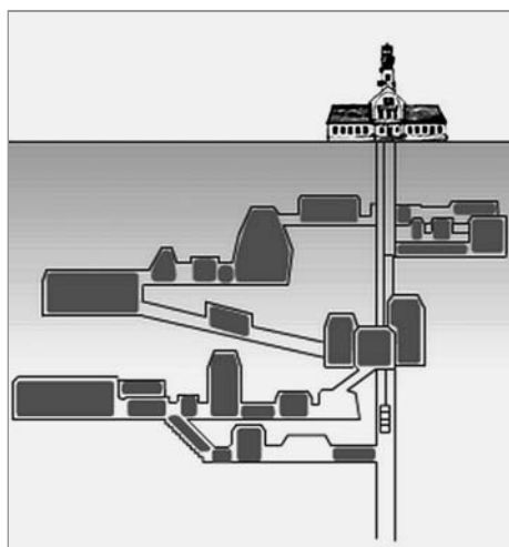
Solný důl Vělička – schéma podzemních prostorů
